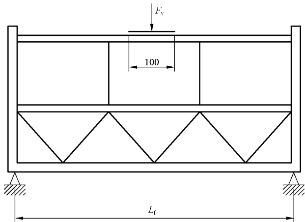
图 A.5 护栏上的垂直载荷
