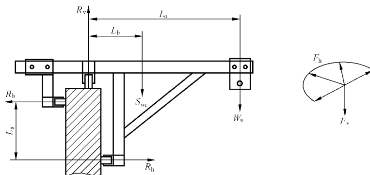
图 11 女儿墙卡钳
