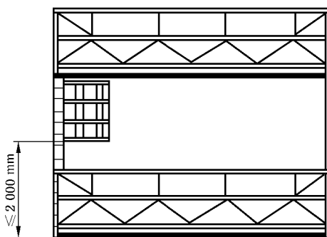
图 14 多层平台
