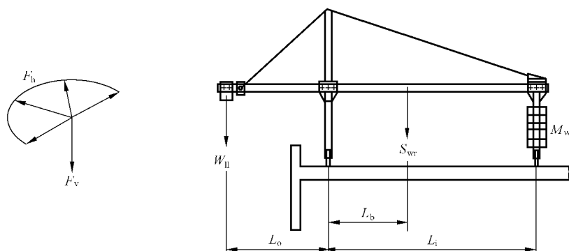
图 12 配重悬挂支架
