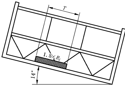
图 A.3 倾斜平台
