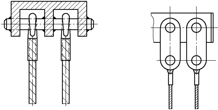
图 16 典型悬挂点示例
