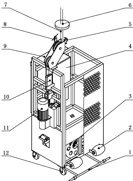
图 2 双吊点平台
