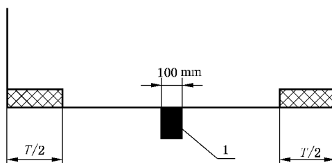
图 9 上升时遇突出物
