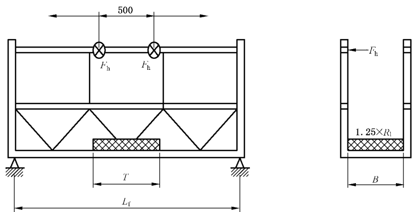
图 A.4 护栏上的水平载荷
